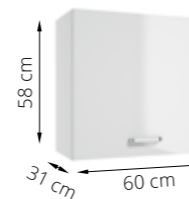
3 FIRST A60 szafka wisząca z 1 drzwiami wall cabinet with 1 door
