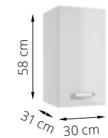
1 FIRST A30 szafka wisząca z 1 drzwiami wall cabinet with 1 door
