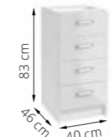
11 FIRST B40 szafka stojąca pod blat z 4 szufladami base cabinet with 4 drawers
